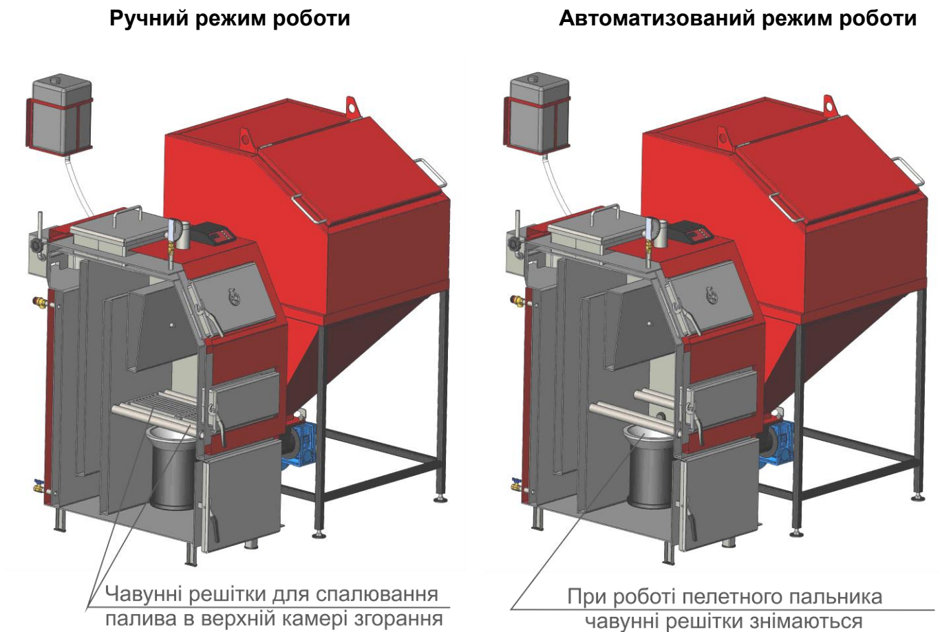
Рис.2 Ручний та автоматизований режими роботи котла
