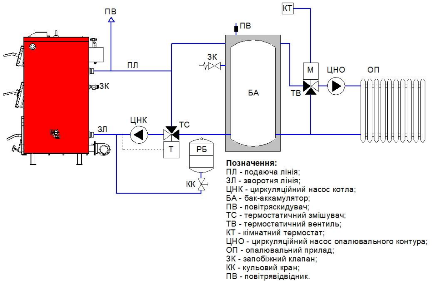
Рис.5 Схема обв'язки котла з баком акумулятором (рекомендована)
