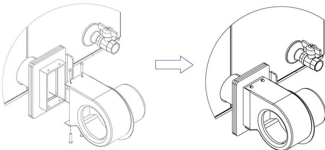
Рис. 12 Схема підключення вентилятора
