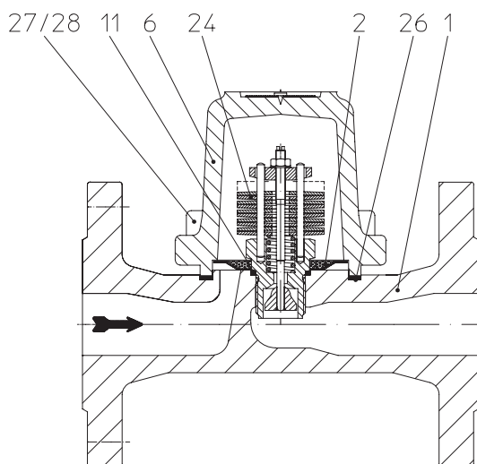
Рис. 1: CONA®B - BR600 PN16 DN15-50
