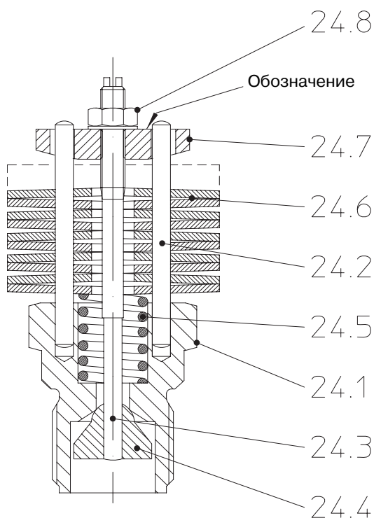
Рис. 10: Бимет. регулятор PN16-100
