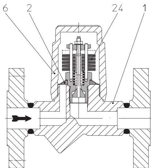
Рис. 2: CONA®B - BR600 PN40 DN15-25
