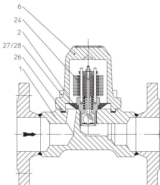
Рис. 3: CONA®B - BR600 PN40 DN32-50
